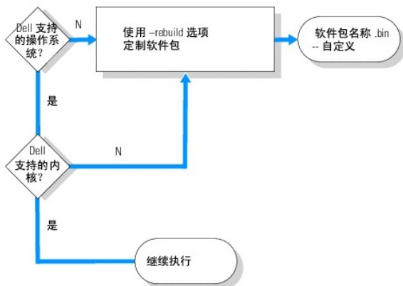
图 4-1. 用于重建软件包的 Dell 启用途径
